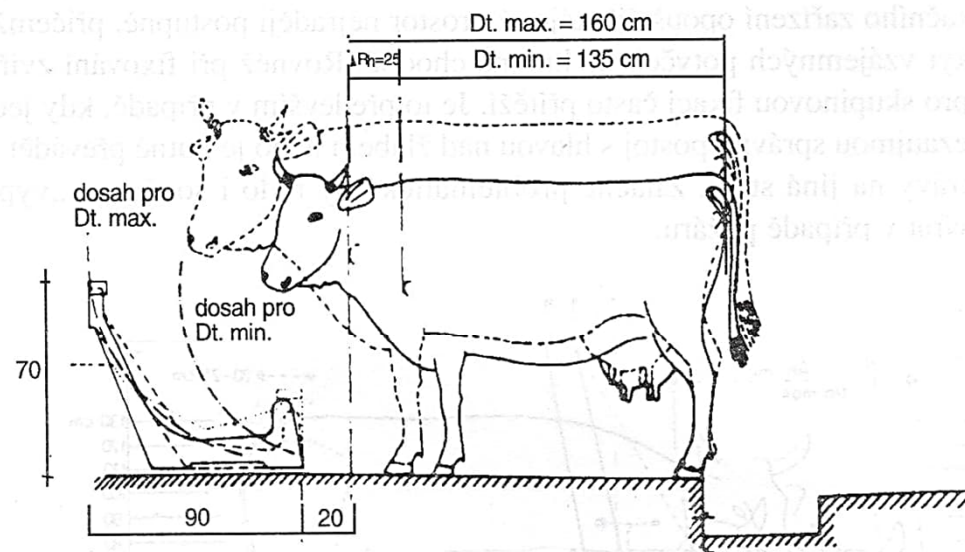
Obr. 13: Rozdílné dosahy při příjmu krmiva nejmenšími a největšími kravami na stání odpovídajícímu největším zvířatům při postavení zadních končetin na konci stání (18)
