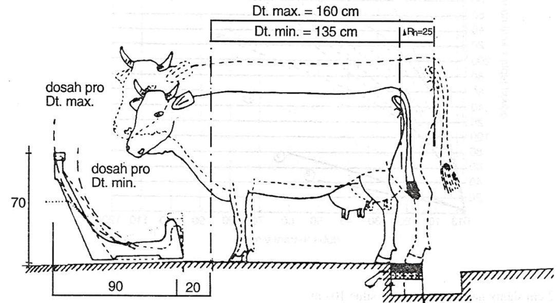
Obr. 14: Nutné rozdíly v délce stání při stejné poloze fixačního zařízení pro největší a nejmenší krávy (18)
