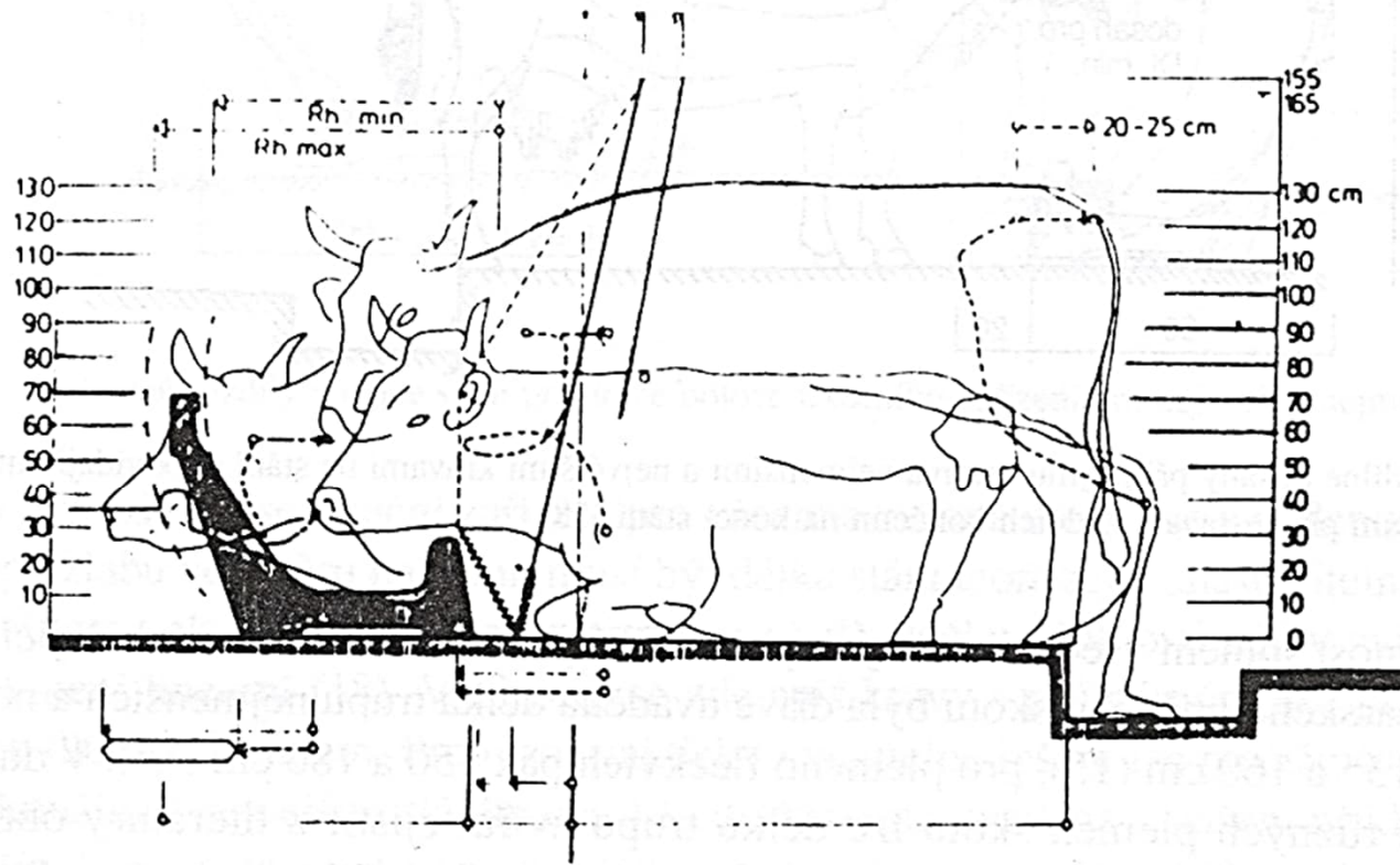
Obr. 12: Krátké stání s krmným stolem a kloubným fixačním zařízením umožňuje přirozené vstávání (13)
